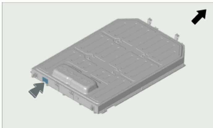
Заводская табличка с информацией о продукте аккумуляторной батареи наклеена на внешней стороне тягового аккумуляторного блока.
