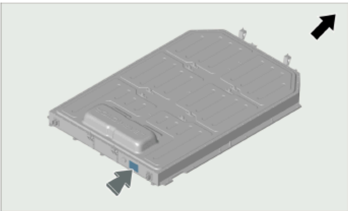
Предупреждающая надпись о высоком напряжении наклеена на внешнюю сторону тягового аккумуляторного блока.
