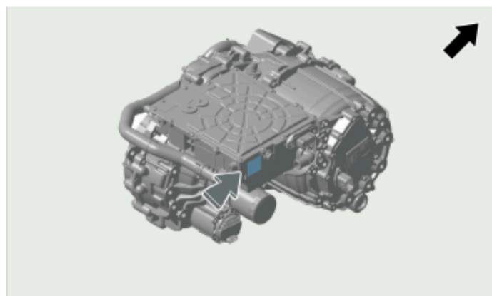
Предупреждающий знак о высоком напряжении и ручной знак предупреждения о поражении электрическим током расположены на корпусе блока управления двигателем.
