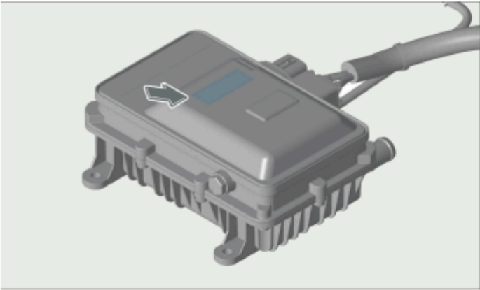
Водонагреватель РТС (состояние II) с предупреждающей надписью HV наклеен на поверхность водонагревателя РТС.
