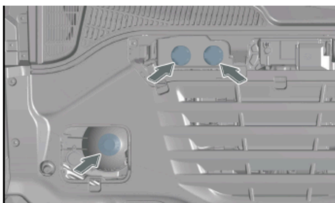
Предупреждающая надпись о охлаждающей жидкости наклеена на крышку расширительного бачка для охлаждающей жидкости.
